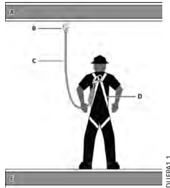
Fig. 7 - Detención de caídas (PFAS)
