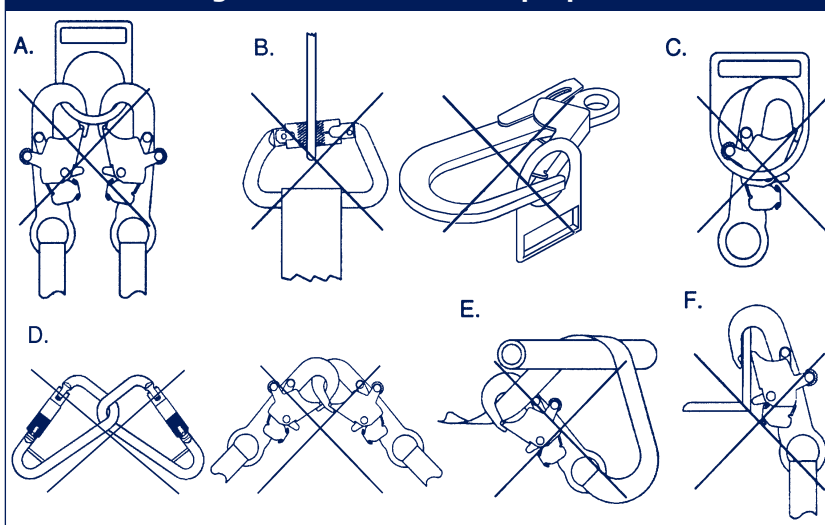
Figura 3: Conexiones inapropiadas
