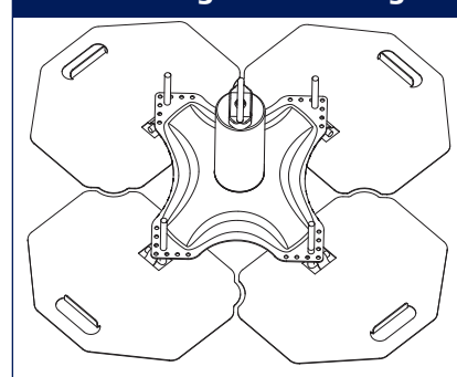
Figure 10 - Assurer l'emboîtement de l'ancrage
